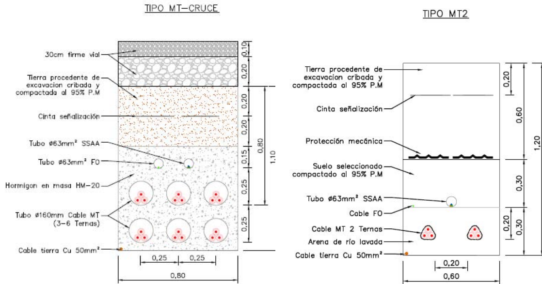
Ilustración 3: Zanjas MT
